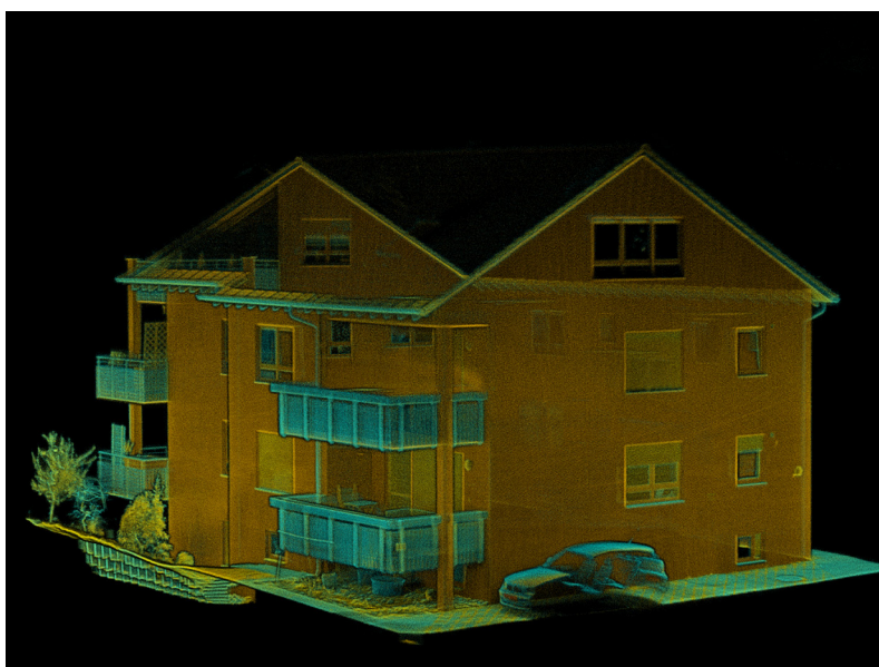
Acquisizione di una nuvola di punti con Scanner LiDAR per determinare le superfici e le quantità per la facciata esistente.
