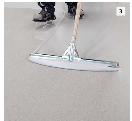
3 Come sigillante coprente colorato su rivestimenti sabbati per pavimentazione industriale antiscivolo
