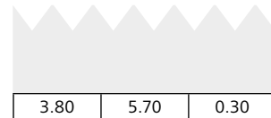
Zahnform 92
