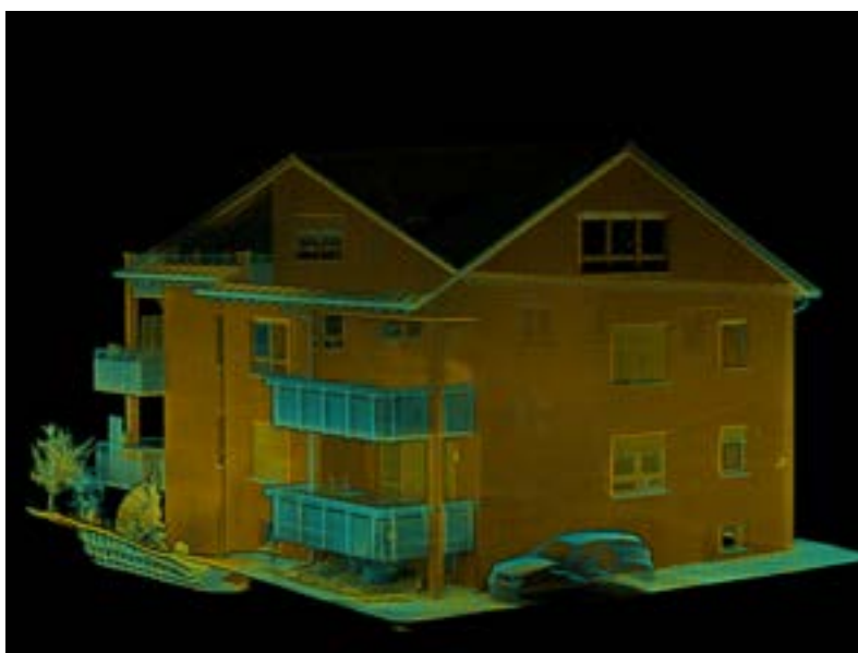
Acquisition d'un nuage de points à l'aide d'un scanner LiDAR pour calculer les surfaces et les volumes de la façade existante.
