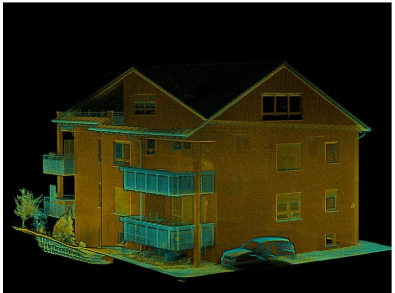
Aufnahme einer Punktwolke mittels LiDAR-Scanner zur Ermittlung von Flächen und Mengen der Bestandsfassade.
